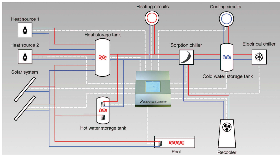
◀ Abbildung 2 Systemschaubild chillii® Solar Cooling System mit chillii® System Controller HC
