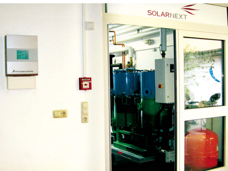
◀ Abbildung 3 chillii® System Controller HC und Absorptionskältemaschine chillii® ESC15 des solaren Kühlsystems der Hightex GmbH
